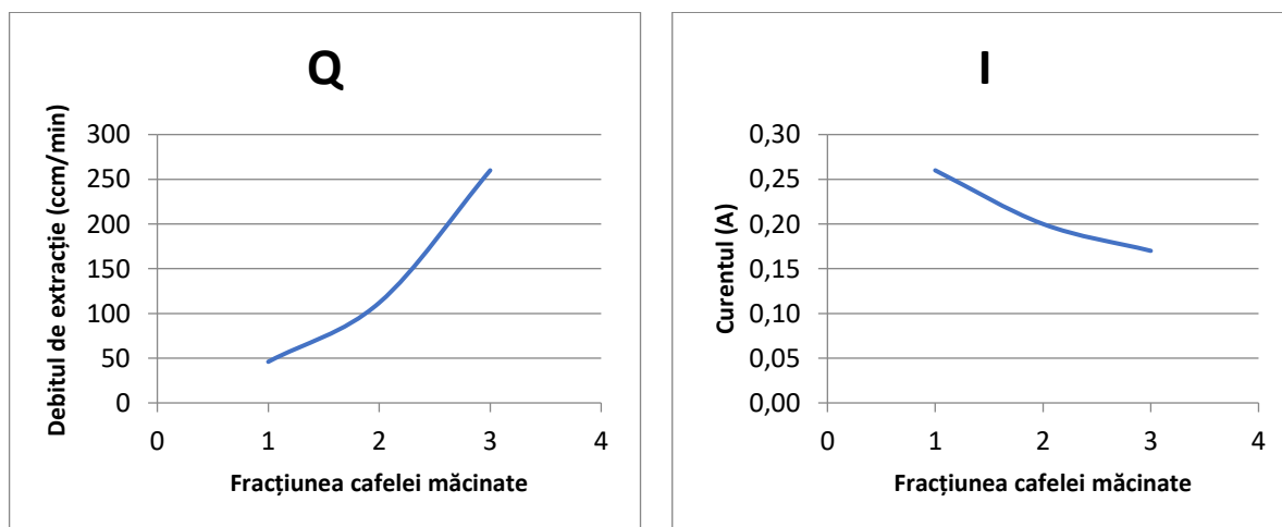
Fig. 2.4. Dependenta debitului și curentului în funcție de fracția de cafea [elaborat de autor]
