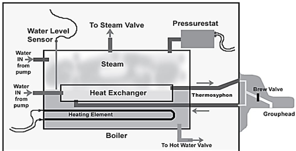
Fig. 1.16. Diagrama de reprezentare a boilerului multi-sețiunat al aparatului de cafea VIBIEMME DOMOBAR SUPER [18]
