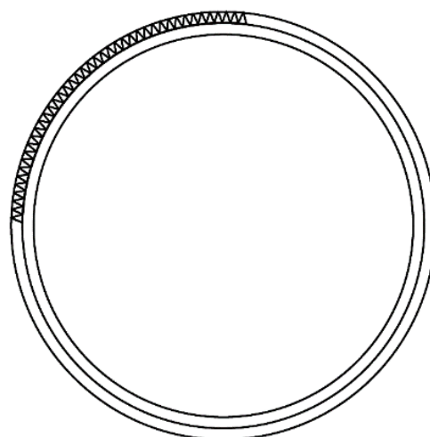
Fig. 3.16. Roata dințată a sistemului de ajustare automatizată [elaborat de autor]
