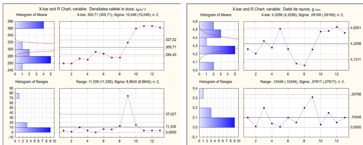
Fig. 2.21. Analiza SixGraph X-bar și R Chart pentru densitatea de cafea în doză tasată corespunzătoare debitului de răsnire. [elaborat de autor]
