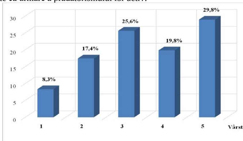
Fig. 3.10. Structura de vârstă a speciei Lepomis gibbosus din lacul refrigerent Cuciurgan
