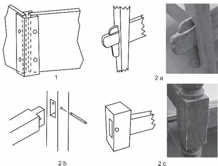
Fig.2.34. Sisteme de asamblare utilizate la confecționarea paturilor: 1- îmbinarea în „pană și uluc”; 2, a – îmbinare cu „cep și scobitură” - îmbinarea liberă cu pană; 2, b, c – îmbinarea cu „cep și scobitură”- îmbinare deschisă. Desene Elena Madan. Foto Aida Bondari (2020).
