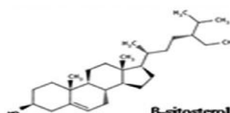
β-sitosterol
