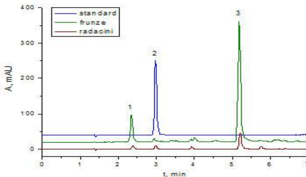
Figura 5. Cromatogramele obținute la analiza materiei prime de pădăie.
