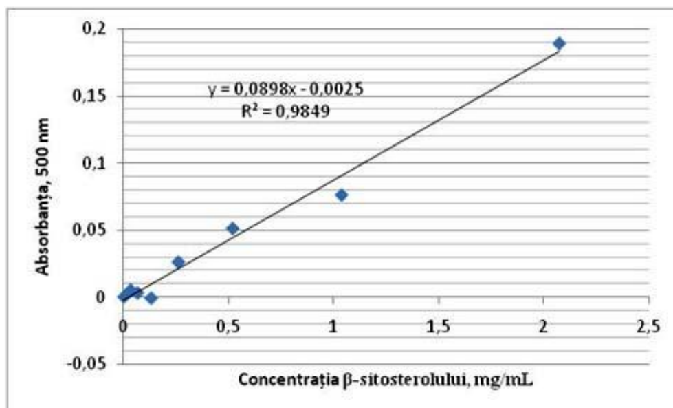
Figura 4. Curba de calibrare a \beta -sitosterolului, mg/mL.
