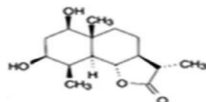
Tetrahydroidentubin
