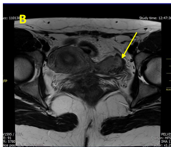
Fig.3.39. IRM, în ponderație T2, plan axial. Uterul unicorn pe dreapta (A) cu corn rudimentar noncomunicant cavitar pe stângă (B), cavitatea endometrială a cornului rudimentar este micșorată în volum
