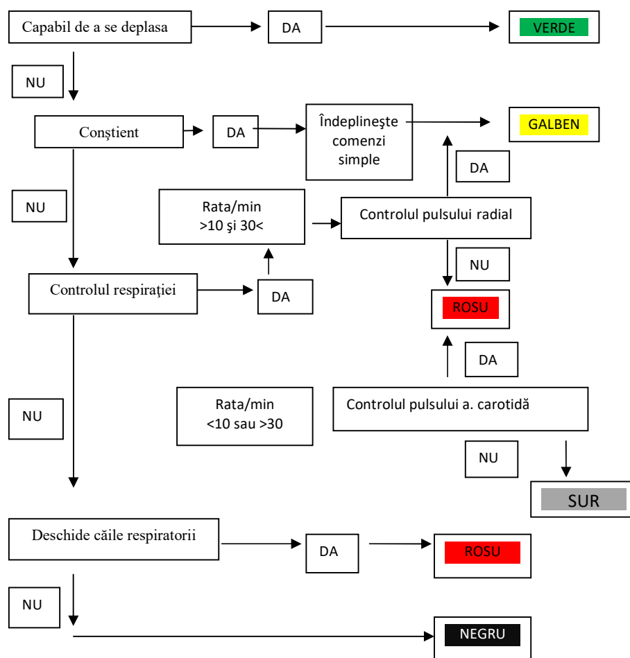
Figura 3. Algoritmul TRAMIN
