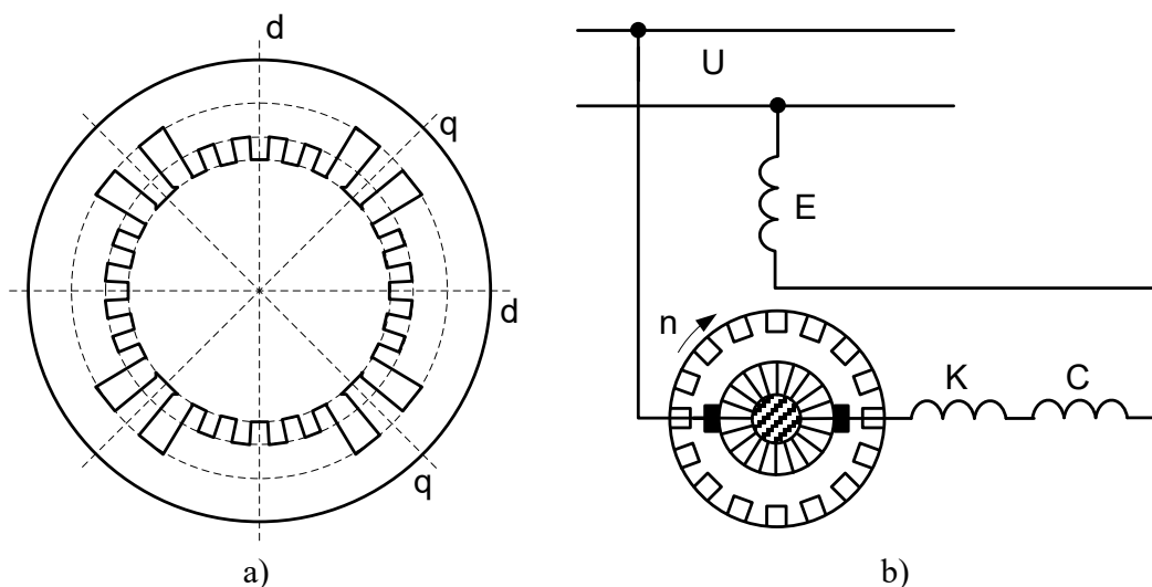
Fig. 1.18. Mașina monofazată cu înfășurare de excitație serie: a) tolă statorică la mașina monofazată serie; b) schema electrică a mașinii monofazate serie.
