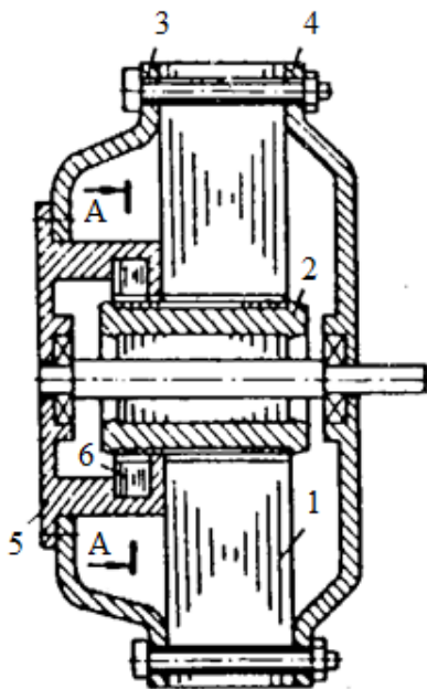
Fig. 1.14. Schema constructivă a motorului asincron monofazat.
