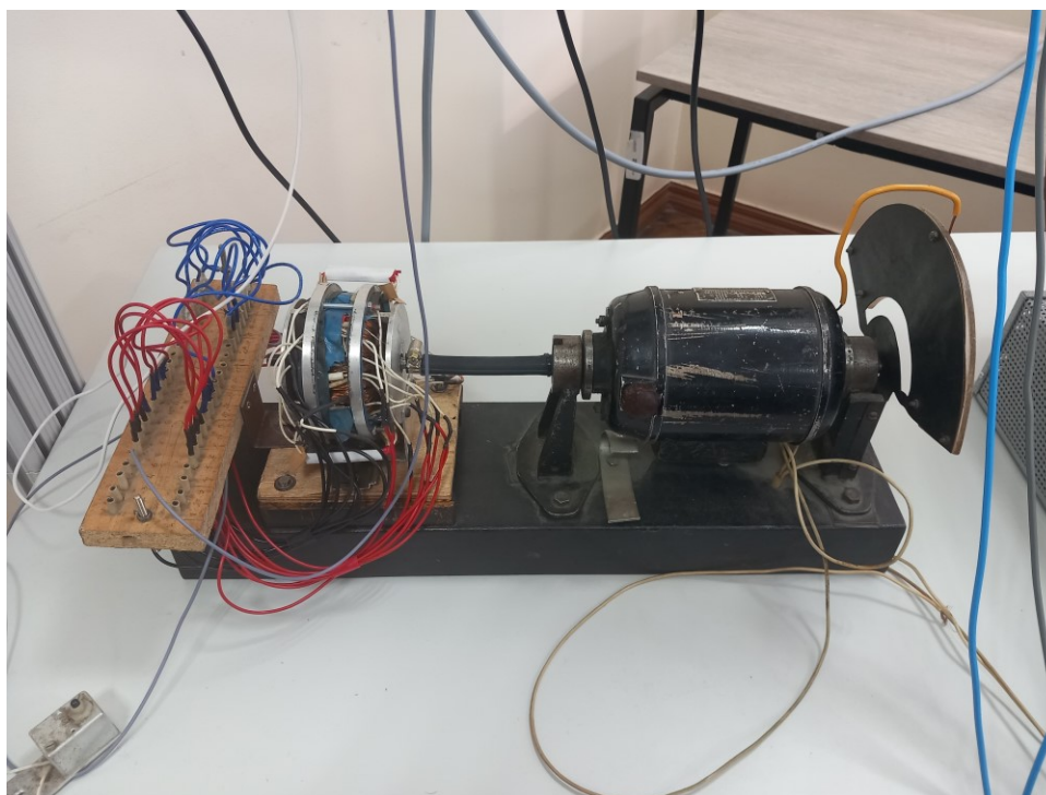
Fig. 4.10. Grupul motor-frână pentru încercarea în regim de sarcină.
