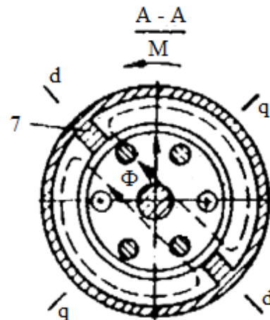
Fig. 1.15. Secțiunea A-A.
