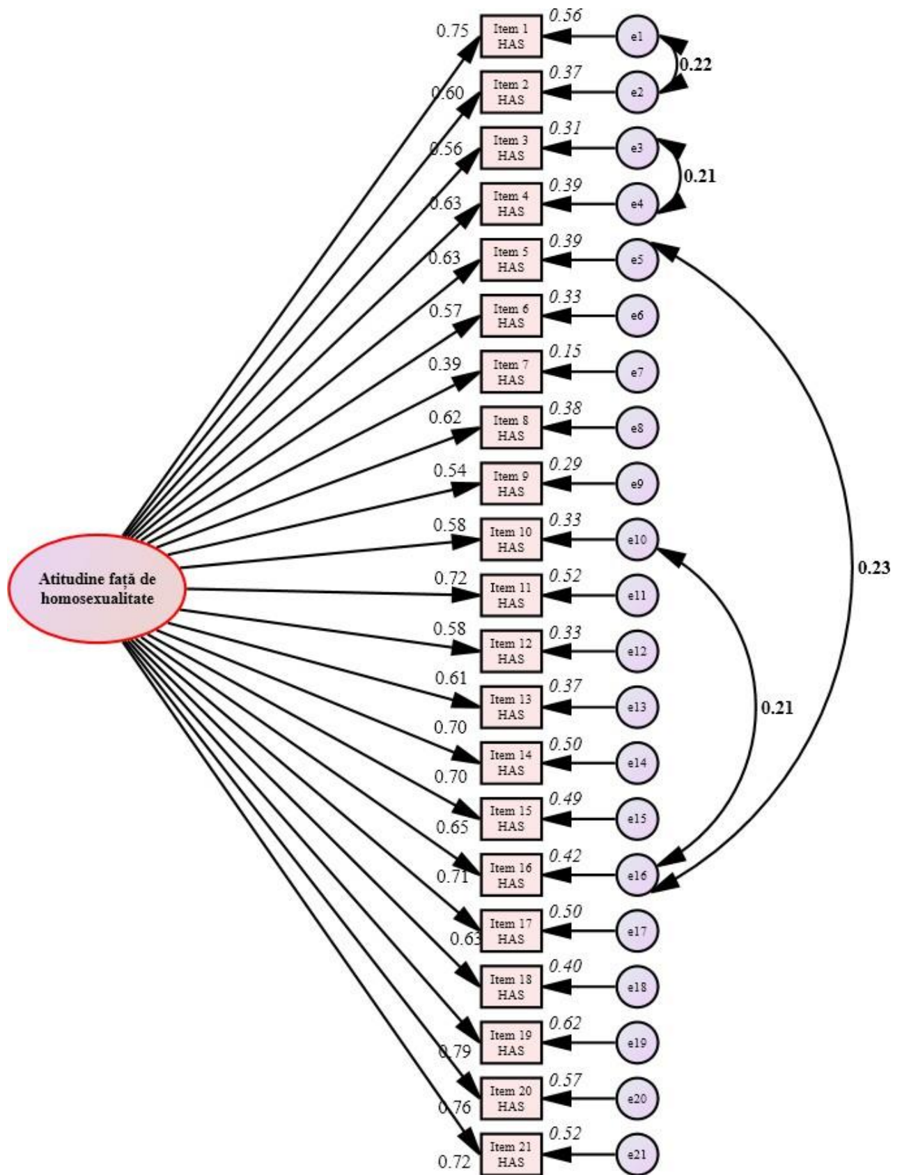
Fig. A4.1. Modelul metric final pentru versiunea în limba română a instrumentului HAS
