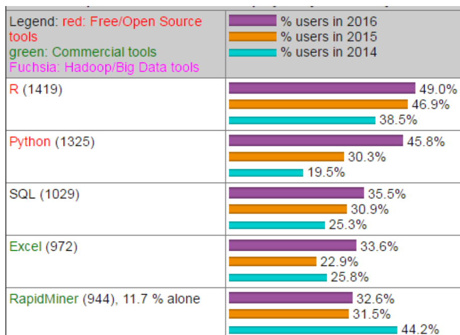
Figura 1.6. Analiza comparativă a software Data Mining 2014-2016 [93]
