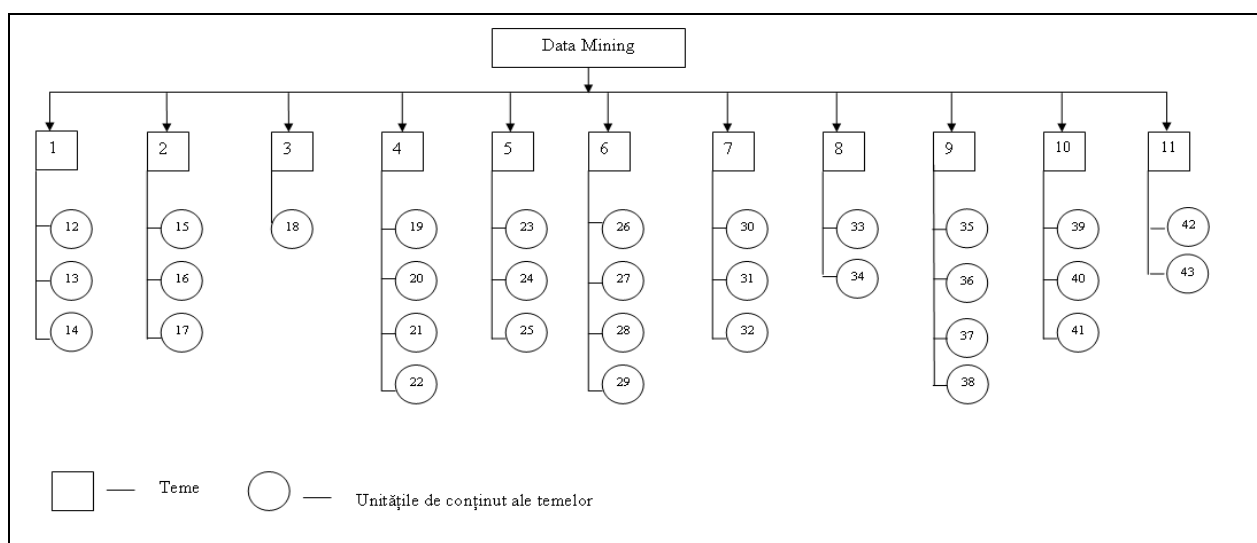
Figura 2.3. Graful de prezentare a conținutului cursului „ Data Mining ”
